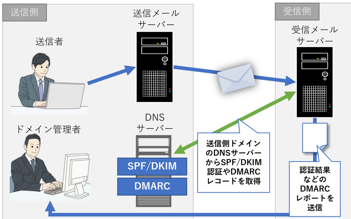
図表3-2-11 DMARC レポートの送信
