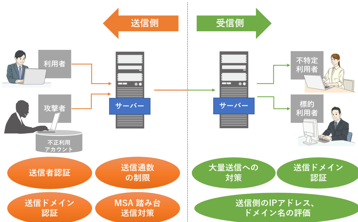
図表 3-2-1 主な技術的な対策の概要
