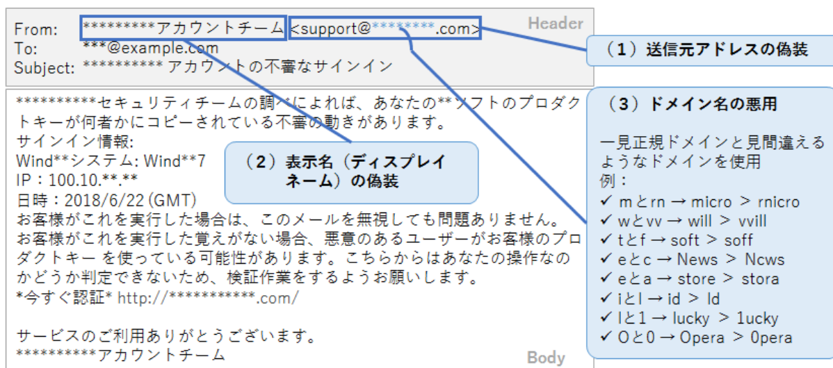
図表 2-4-1 送信元の偽装
